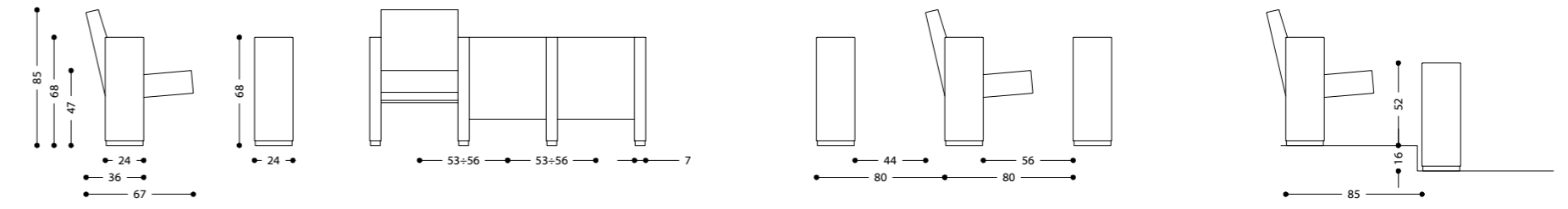
Mura "A" su barra con piede centrale - Mura "A" on beam with central base
