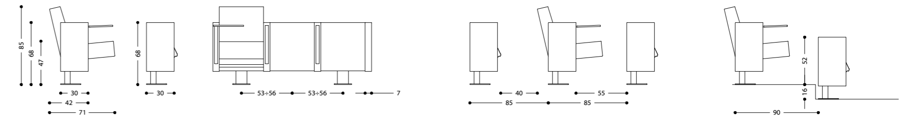
Mura "B" su barra con piede centrale - Mura "B" on beam with central base
